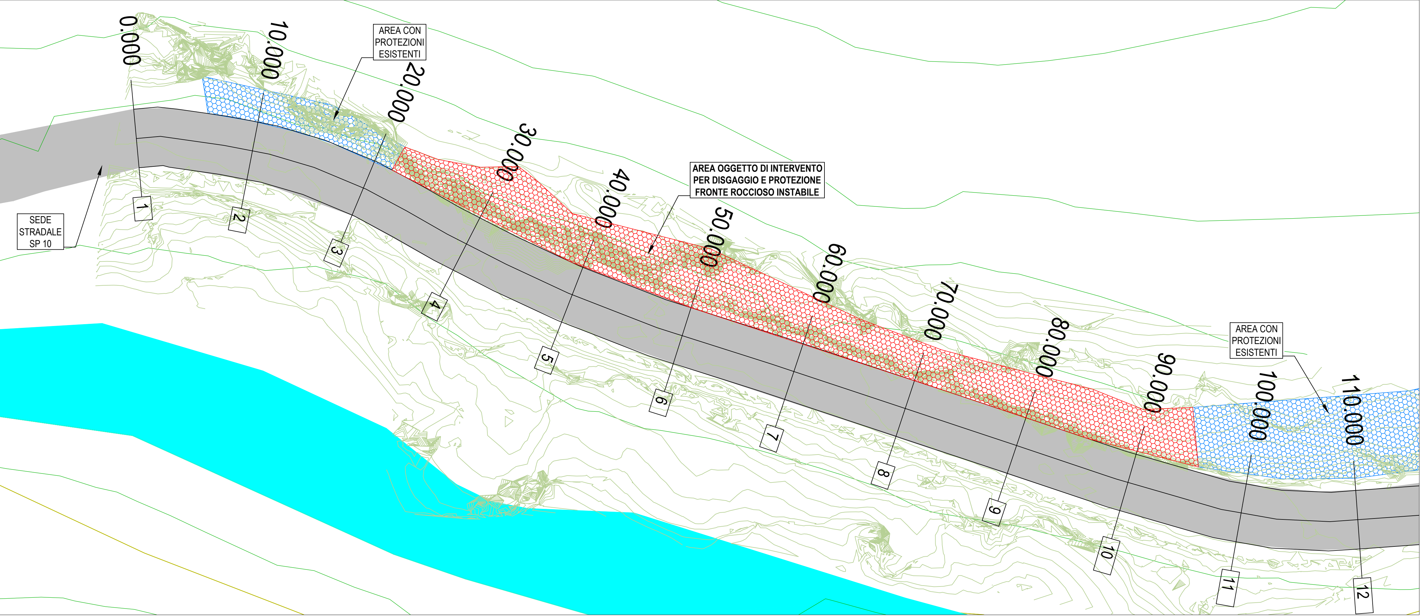
PIANTA DI PROGETTO SCALA 1:250
